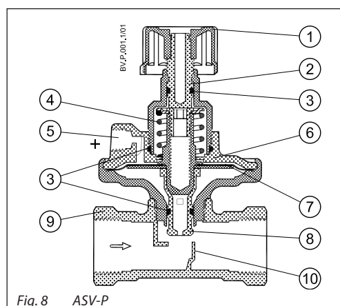
Fig. 8 ASV-P
