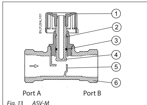
Fig. 13 ASV-M
