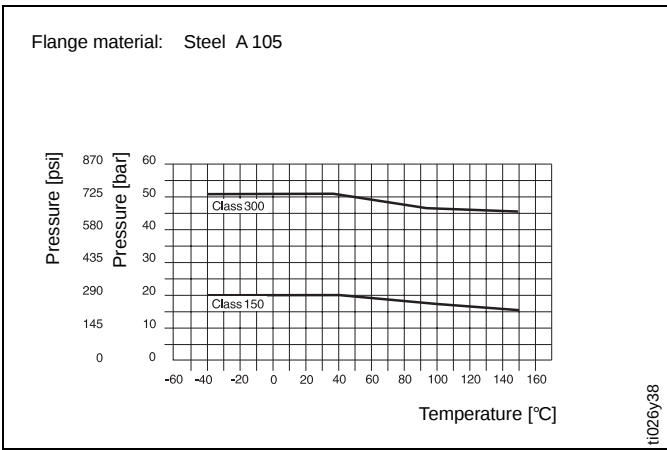
Promag F (ANSI B16.5)
